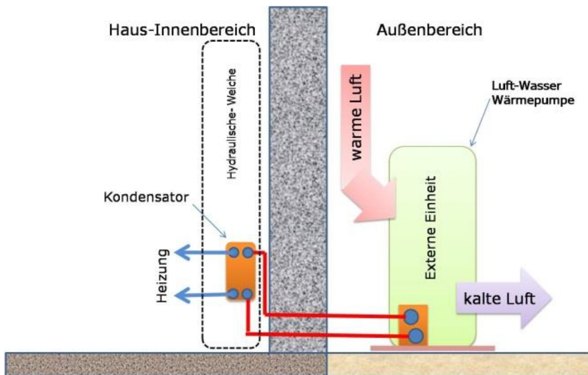
Abbildung 1 zeigt das Schema einer Luft-Wasser Wärmepumpe
