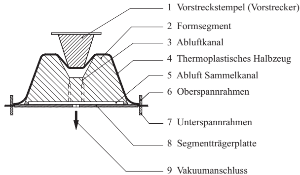
Bild 1.1 Prinzipskizze Warmumformen
