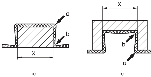
Bild 2.1 Positiv- und Negativformung a) Positivformung (schematisch) b) Negativformung (schematisch) X = vom Formwerkzeug abgeformtes Maß
