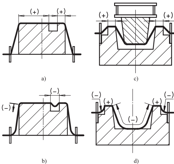
Bild 2.3 Schematische Darstellung des resultierenden Ausformdrucks als Summe von Umform- und Rückstellkraft eines Halbzeugs
