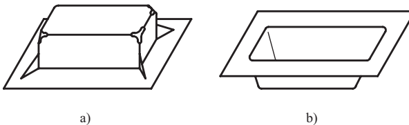
Bild 2.2 a) Positiv geformtes Teil mit Falten zum Rand und Schreckmarken an den Ecken am Übergang vom Boden zu den Seitenwänden b) Negativ geformtes Teil ohne Falten und einem ringsum gleichmäßig dicken Rand
