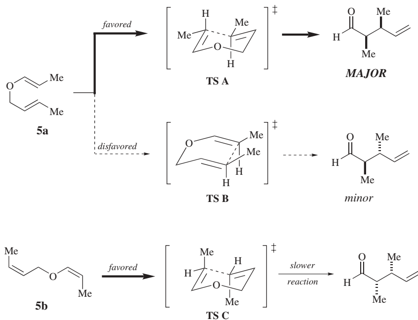
Scheme 1.VI
