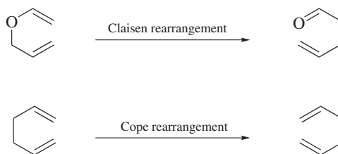
Scheme 1.I
