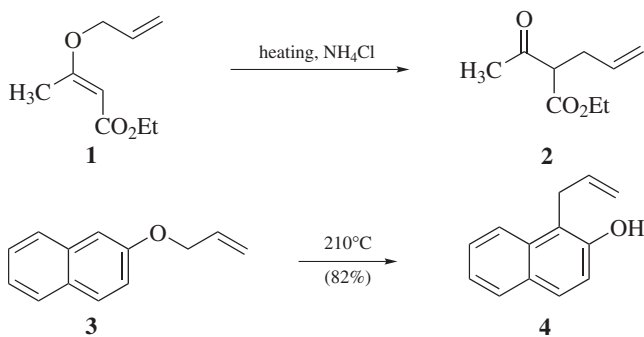
Scheme 1.II
