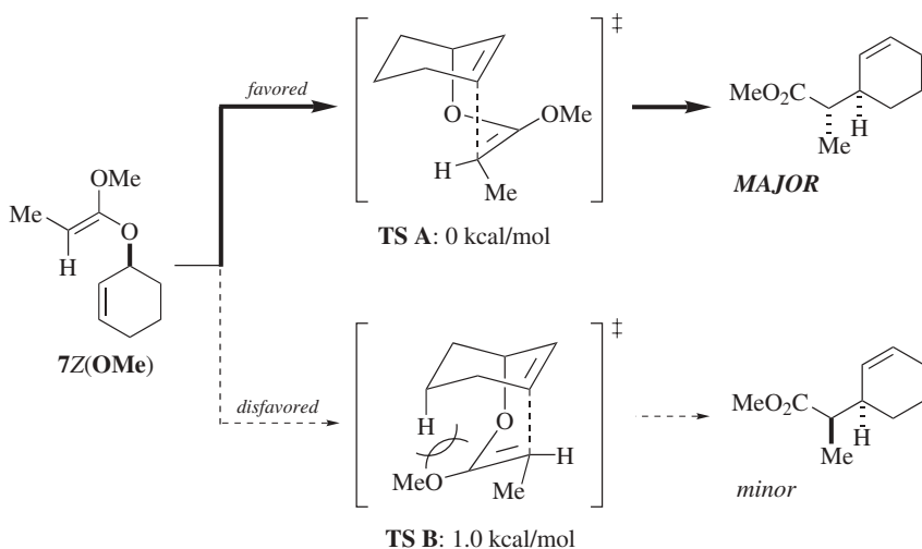
Scheme 1.VIII
