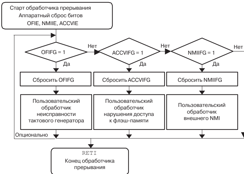
Рис. 2.5. Алгоритм обработки немаскируемого прерывания.
