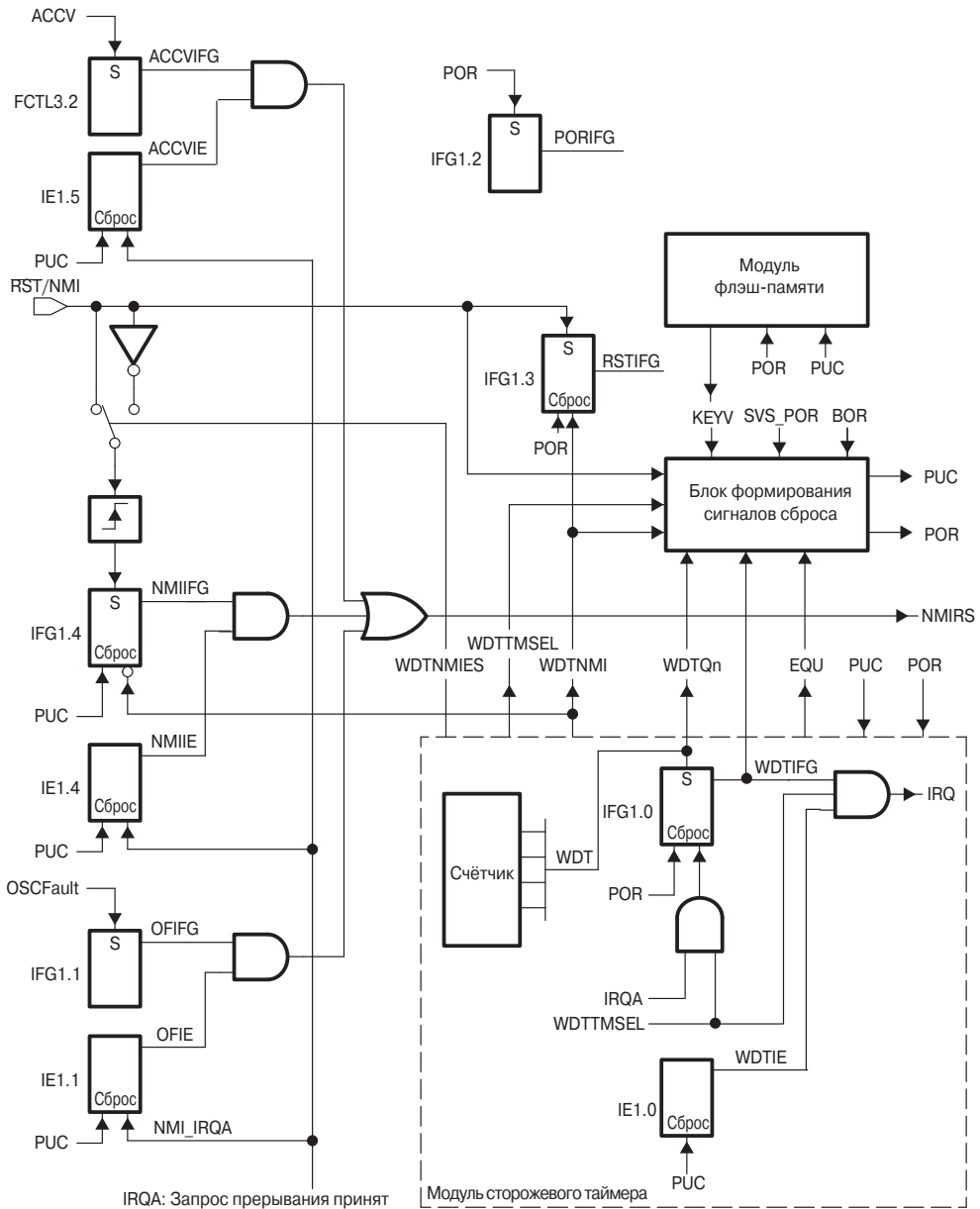
Рис. 2.4. Блок-схема источников немаскируемого прерывания.
