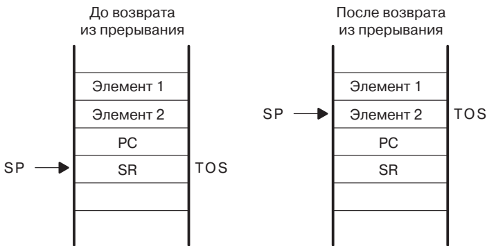
Рис. 2.7. Возврат из прерывания.
