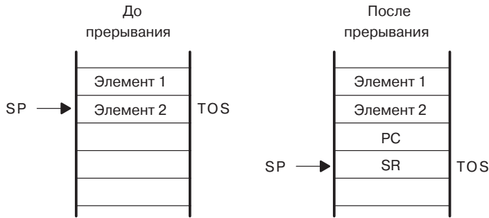
Рис. 2.6. Обработка запроса на прерывание.
