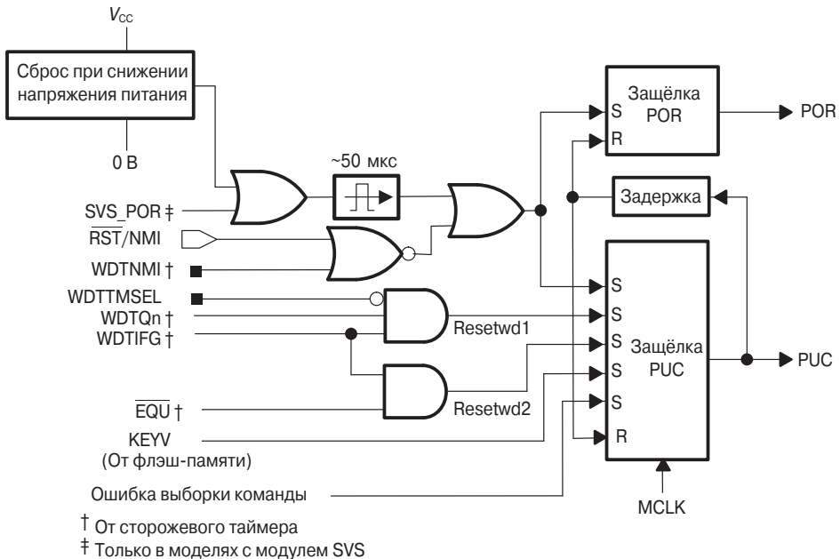
Рис. 2.1. Подсистема сброса.
