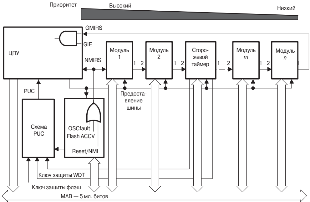
Рис. 2.3. Приоритеты прерываний.
