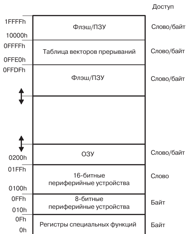
Рис. 1.2. Карта памяти.
