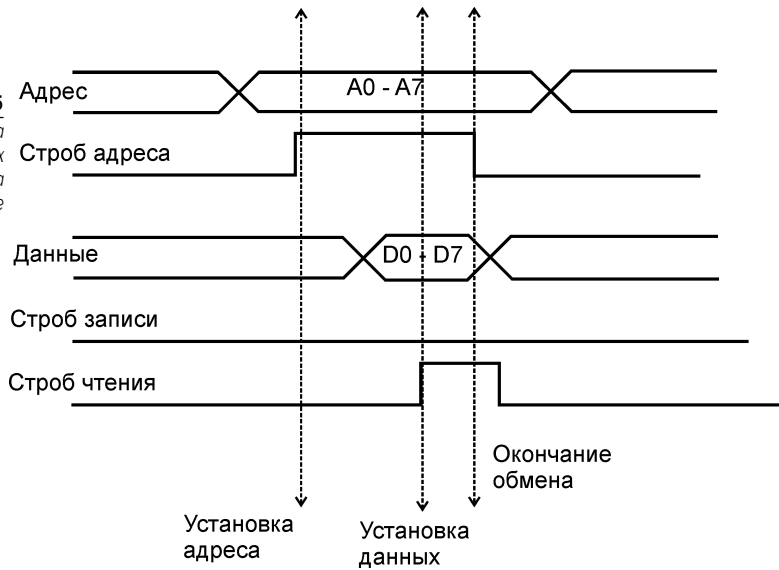
Рис. 2.5 Временная диаграмма чтения данных из устройства на гипотетической шине
