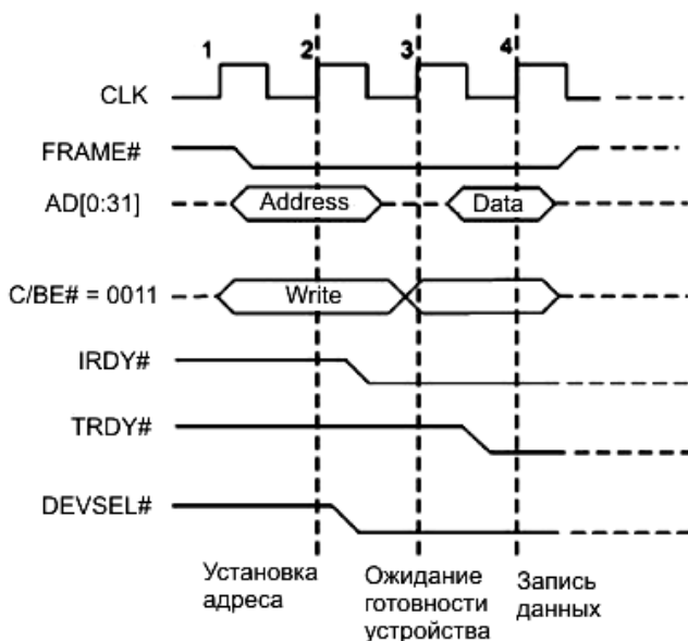
Рис. 2.7 Временная диаграмма работы цикла записи на шине PCI
