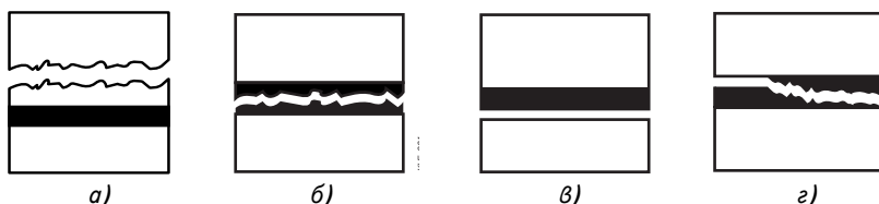
Рис. 2. Характер разрушения клеевого соединения: а и б — когезионный; в — адгезионный; г — на 60% адгезионный и на 40% когезионный
