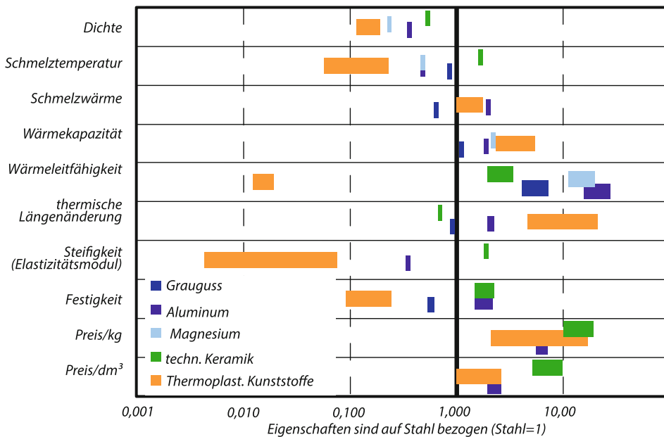
Bild 1.6 Vergleich thermoplastischer Kunststoffe mit Stahl [Bildquelle: WAK-Kunststofftechnik]
