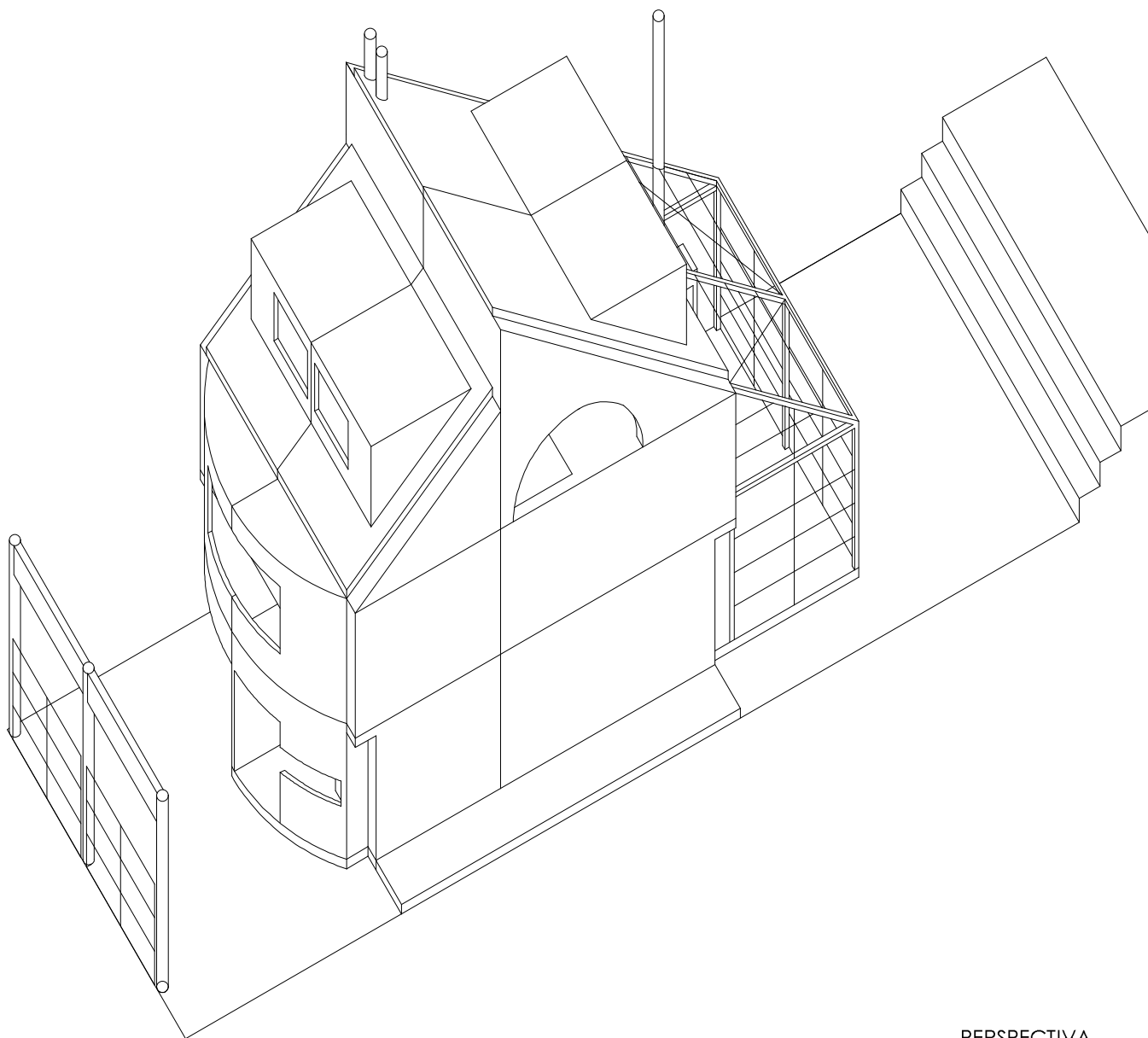
PERSPECTIVA AXONOMETRICA
