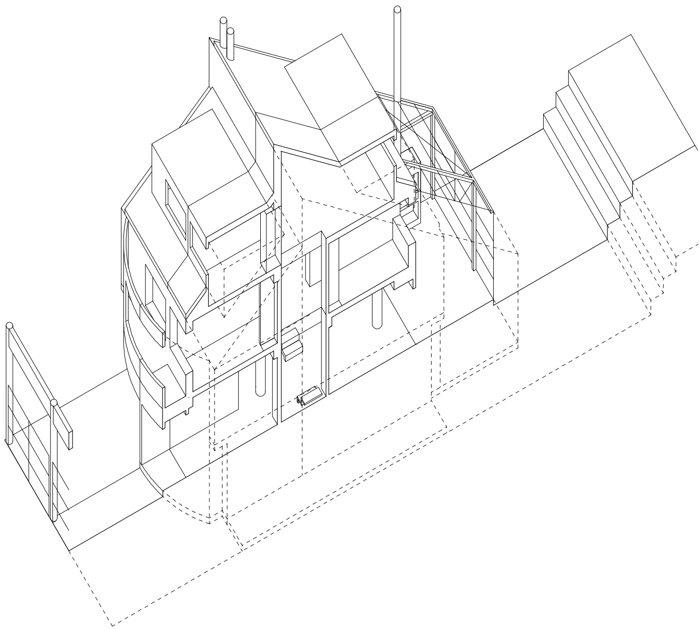
CORTE AXONOMETRICA
