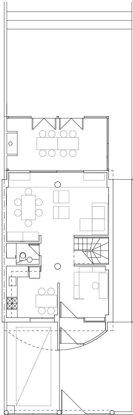
PLANTA BAJA
