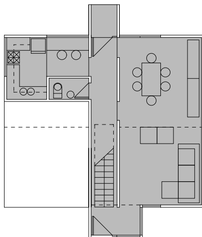
PLANTA BAJA VIVIENDA BASICA
