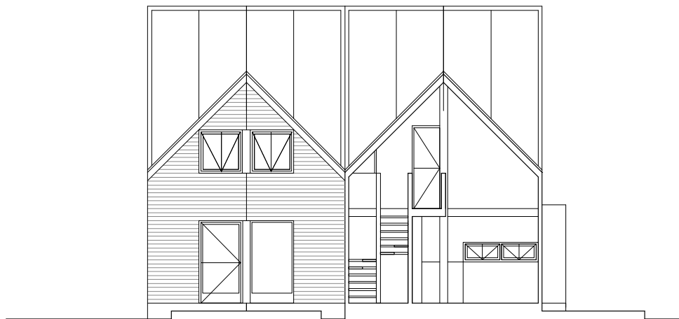
CORTE LONGITUDINAL
