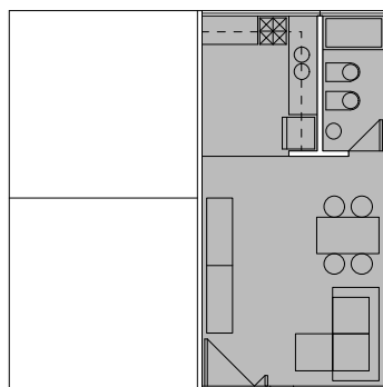
PLANTA BAJA VIVIENDA BASICA
