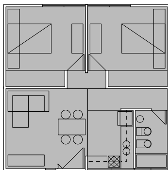
PLANTA BAJA AMPLIACION 2D
