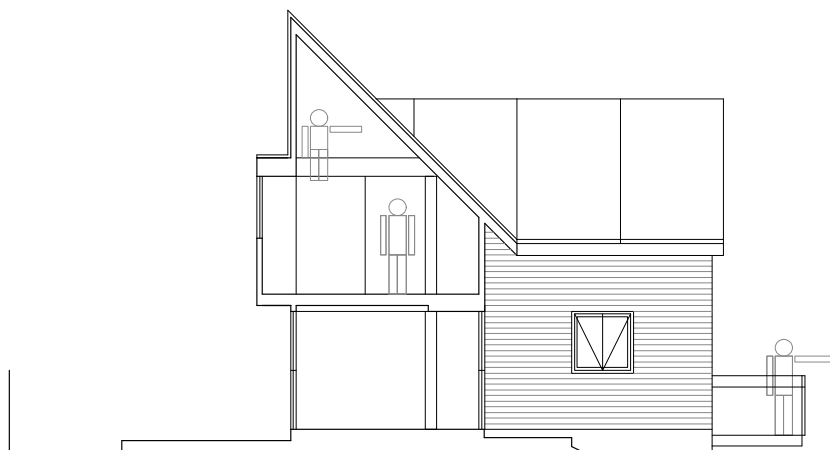
CORTE TRANSVERSAL
