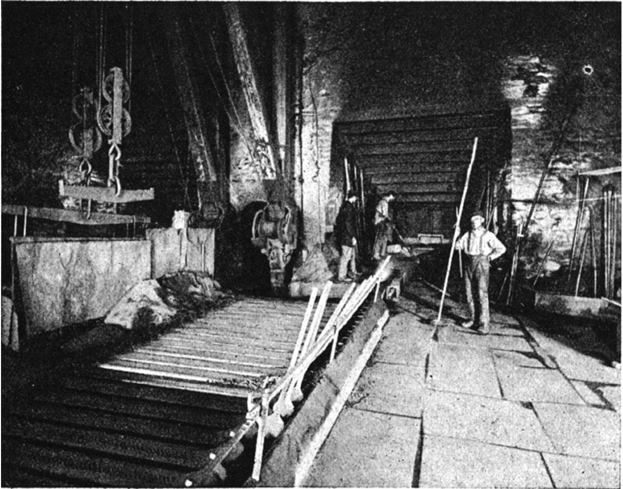
Eine alte Eisenhüttenanlage. Bei dem Dörfchen Rothehütte im Oberharz findet sich heute noch der einzige Hochofen in Mitteleuropa, der noch vollkommen in der Art gehalten ist, wie die Hochofen vor drei Menschenaltern noch allgemein waren. Roteisen und Holzkohle werden mit kleinen Karren in diesen Hochofen gekippt und verhüttet. Foto: Wilhelm Zirkler, Clausthal 1924.
