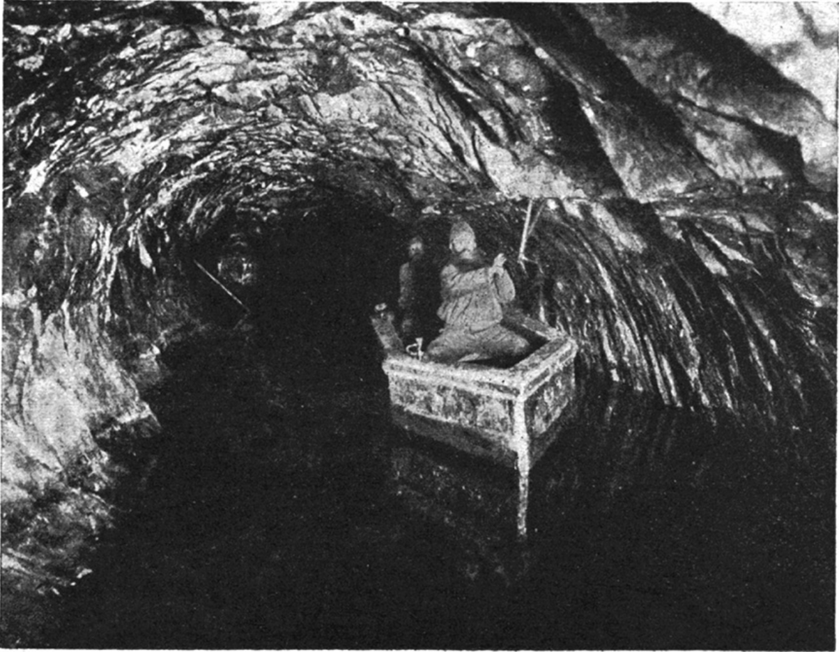
Schiffbare Wasserstrecke unter der Erde (für Artikel über den Ernst-August-Stollen). Solche Stollen sind ursprünglich dazu angelegt worden, um die Wassermengen im Inneren der Erde „zu lösen“. Sie dienen heute noch zur Beförderung von Menschen und Material. Foto: Bormann, Clausthal 1924.
