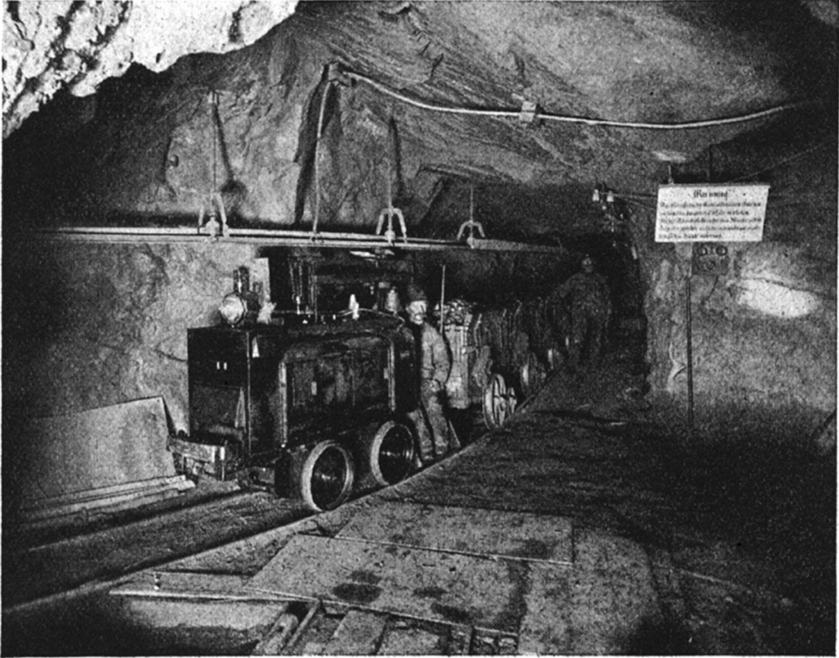
Eine elektrische Kleinbahn, die das gewonnene Erz befördert. Die Tafel rechts warnt vor dem Befahren verbotener Strecken durch Unbefugte und vor dem Berühren der Kontaktschienen. Foto: Wilhelm Zirkler, Clausthal 1924.
