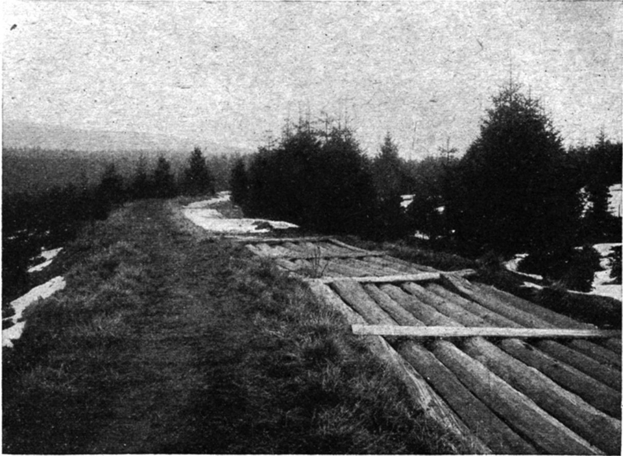
Aufschlaggraben mit Schutzdecke bei Clausthal. Ein ganzes Netz derartiger kunstvoll angelegter Wasserläufe durchzieht den Oberharz und führt den Bergwerken und Aufbereitungsanstalten die zum Antrieb der Maschinen usw. benötigten Wassermengen zu. Foto: Unbekannter Urheber, 1924.
