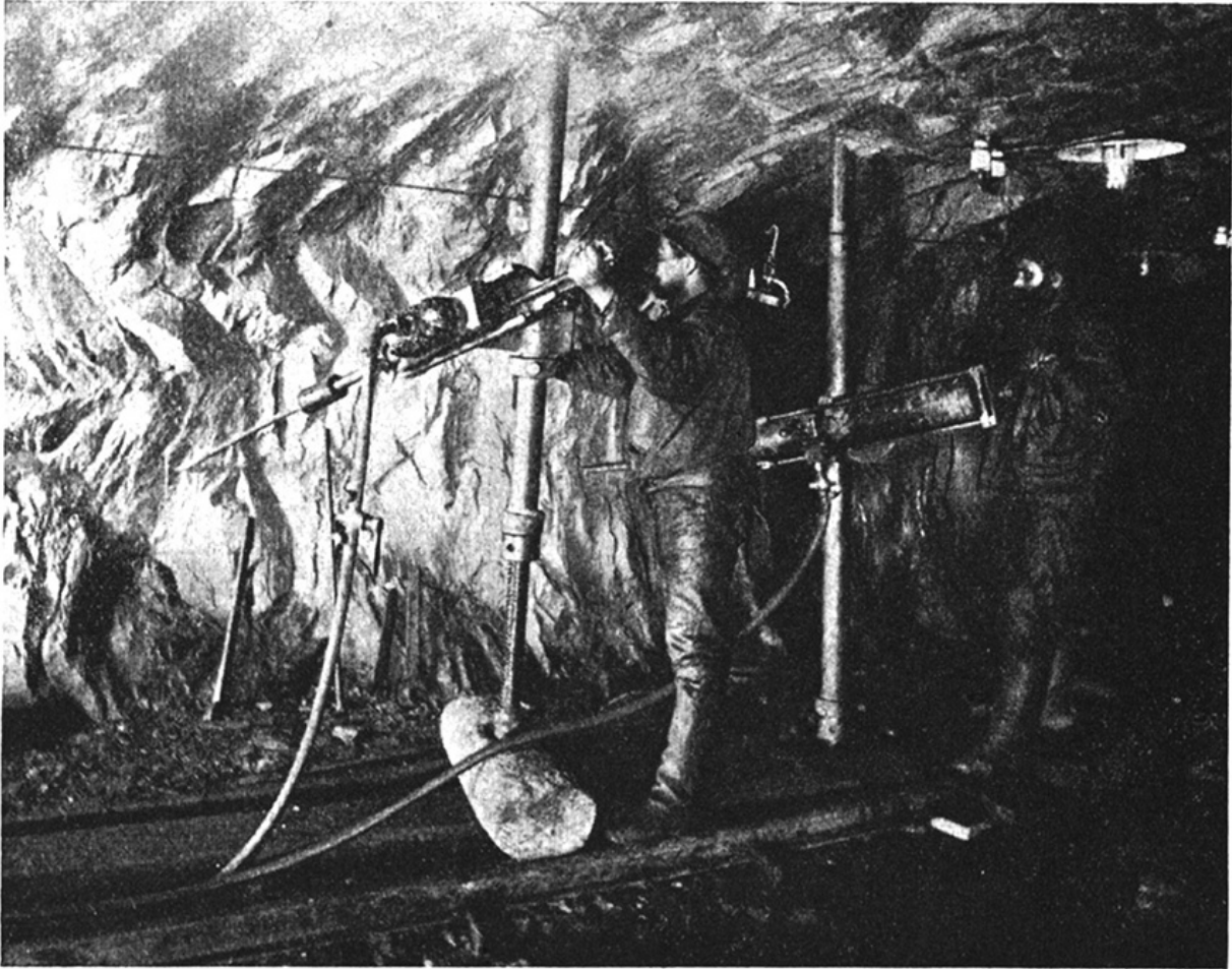
Eine Luftbohr- und eine elektrische Bohrmaschine, die dem Bergmann die frühere Arbeit mit Schlägel und Meißelbohrer abnehmen. Foto: Wilhelm Zirkler, Clausthal 1924.
