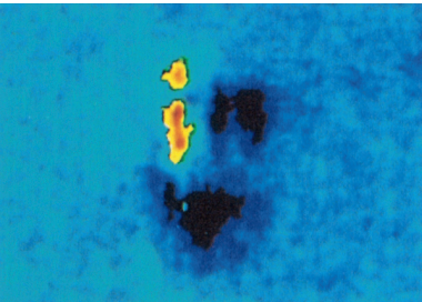
Carga por contacto. Una muestra de plástico de anchura 0,02 mm fue cargada mediante contacto con una pieza de níquel. Aunque el plástico posee una carga neta positiva, se aprecian regiones de carga negativa (oscuras) y regiones de carga positiva (amarillo). La fotografía se tomó barriendo una aguja cargada, de anchura 10^{-7} m, sobre la muestra y midiendo la fuerza electrostática sobre la aguja. (Bruce Terris/IBM Almaden Research Center.)
