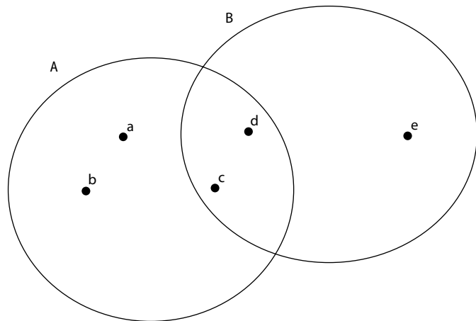
Venn-Diagramm
