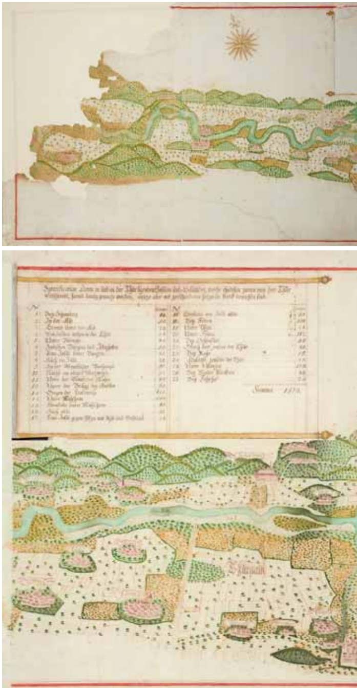
Abb. 2. Die mäandrierende Thur änderte bei fast jedem Hochwasser ihren Lauf, bildete streckenweise mehrere Arme, überflutete die angrenzenden Wiesen, Weiden und Wälder, riss Boden weg und schwemmte neue Kies- und Sandbänke an. Thurkarte von J. B. Sutter (1793). Foto: Winiger (Frauenfeld), Staatsarchiv des Kantons Thurgau [Ausschnitt].
