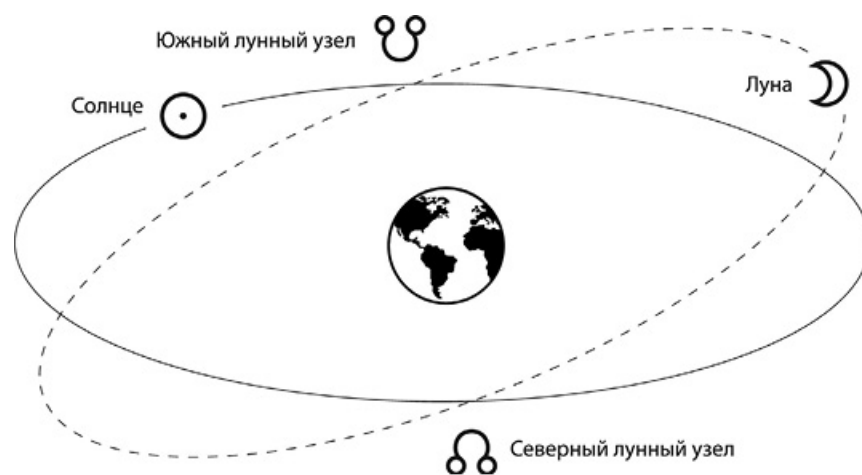
Рис. 1. Пути Солнца и Луны пересекаются в двух точках, образуя лунные узлы
