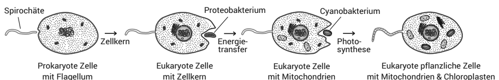
Abb. 2.3. Endosymbiontentheorie. Entwicklung der eukaryoten Zelle aus einer prokaryoten Archaeenzelle durch schrittweise Aufnahme verschiedener Bakterien (Spirochäten, Proteobakterien, Cyanobakterien) als Endosymbionten.
