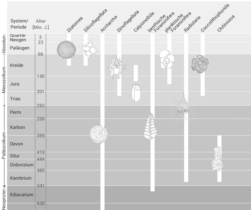
Abb. 2.4. Zeitliches Vorkommen wichtiger Protistengruppen, sowie der Chitinozoen. Bei den Chitinozoen handelt es sich vermutlich um Eigelege vielzelliger wurmförmiger Organismen.
