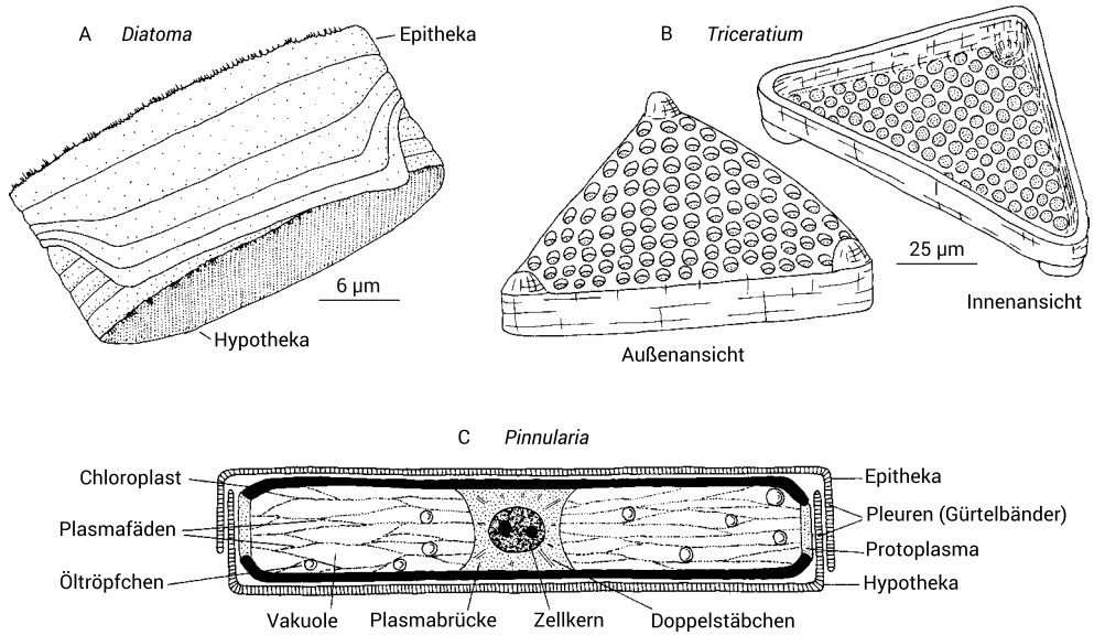
Abb. 2.5. Bau und Skelett der Diatomeen (Kieselalgen) mit Deckel (Epitheka) und Boden (Hypotheka). A: Miozän-rez.; B: Kreide-rez.; C: Oligozän-rez., schematisch. Aus Ziegler (1983a), Abb. 29.
