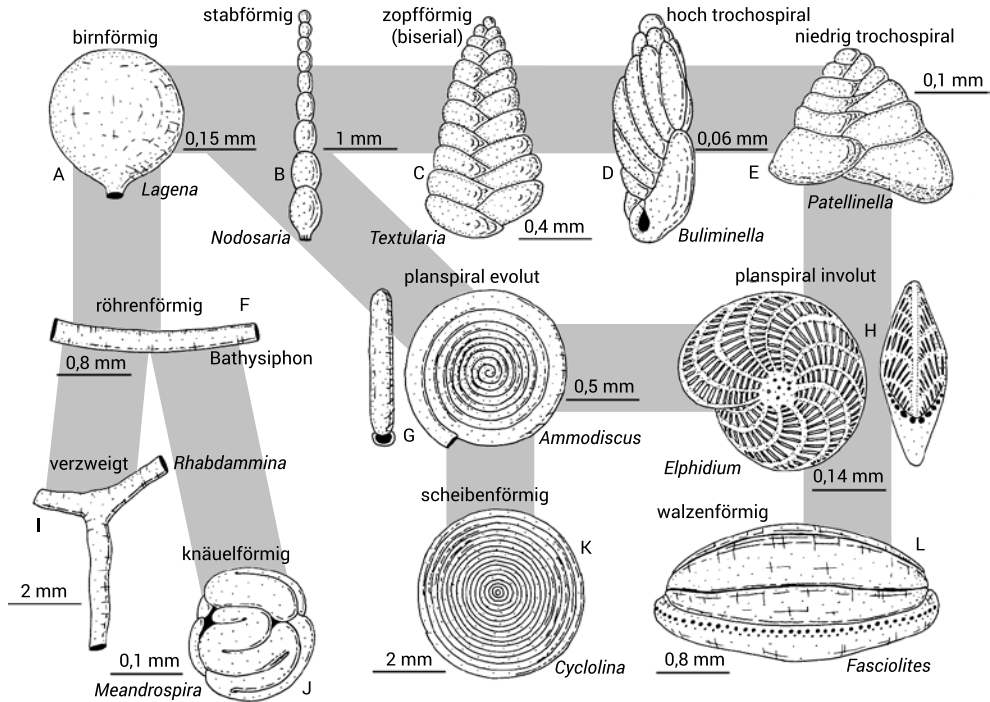
Abb. 2.10. Verschiedene Gehäuseformen bei Foraminiferen (Lochschalen-träger). A: Jura-rezent; B: Perm-rezent; C: Karbon-rezent; D: Kreide-rezent; E: rezent; F: Kambrium-rezent; G: Silur-rezent; H: Eozän-rezent; I: Ordovizium-rezent; J: Perm-rezent; K: Kreide; L: Paläozän-Eozän. Aus Ziegler (1983a), Abb. 39.
